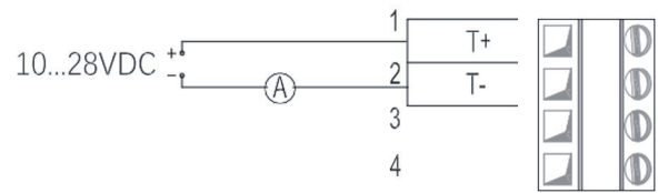
TR13单温变送器电流输出型接线（2线制）
