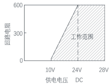
TR13供电电压和回路电阻关系
