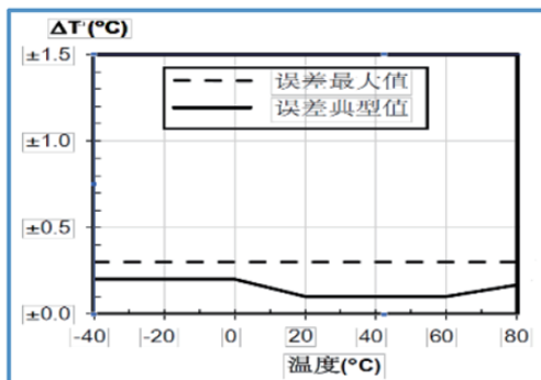
图 1 温度检测误差分布
